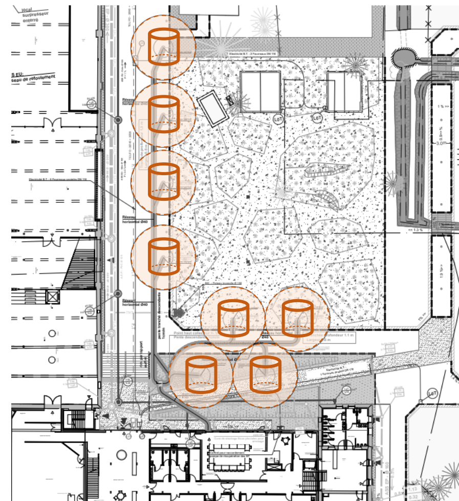
Installation des 8 sondes géothermiques
