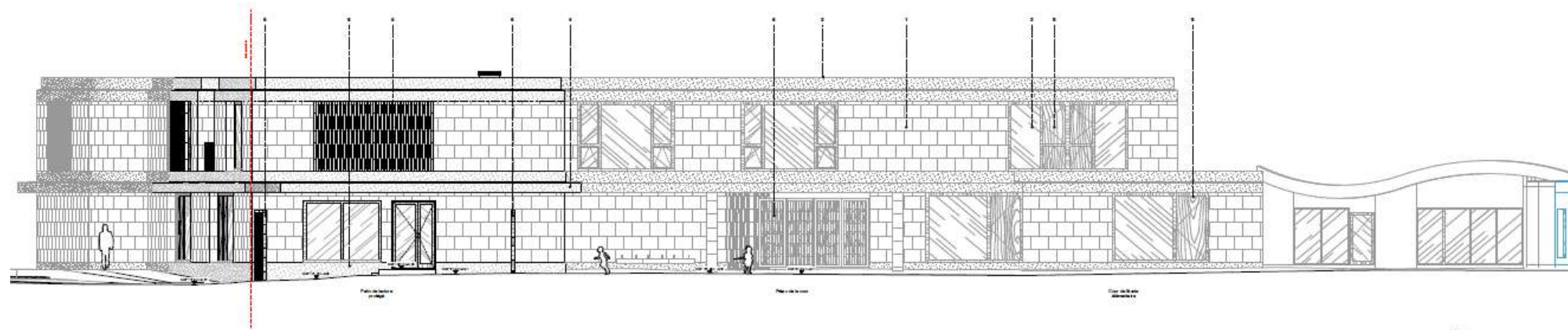
Façade Nord
