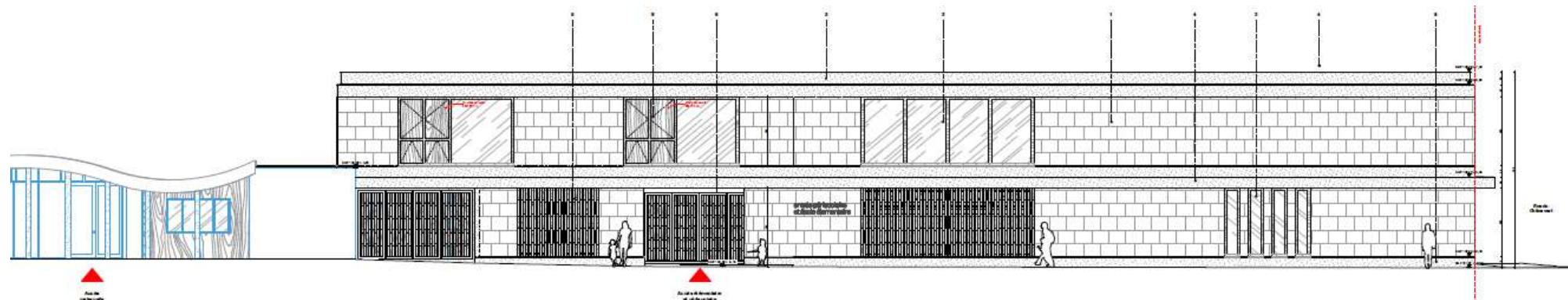
Façade Sud
