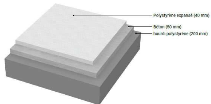
Plancher bas sous VS
