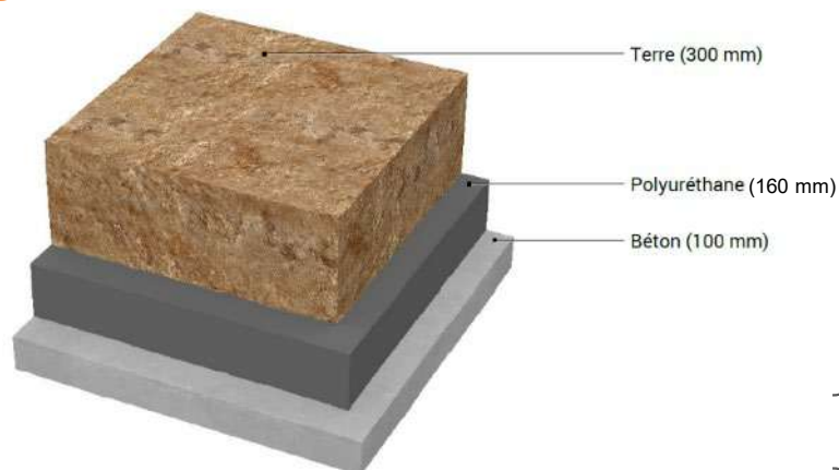
Plancher Haut (végétalisé)
