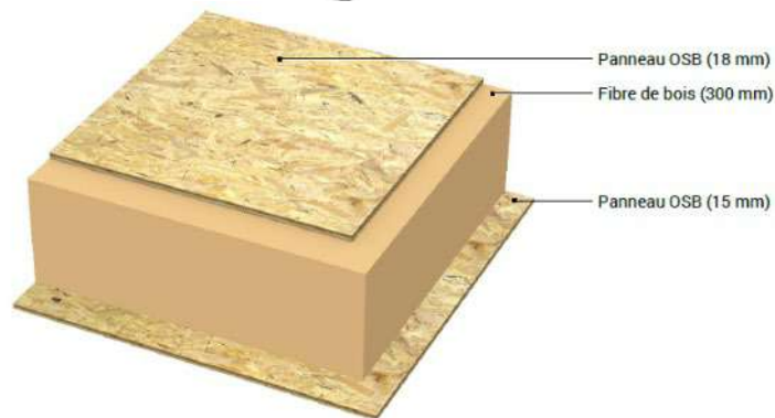
Plancher Haut (Dôme)
