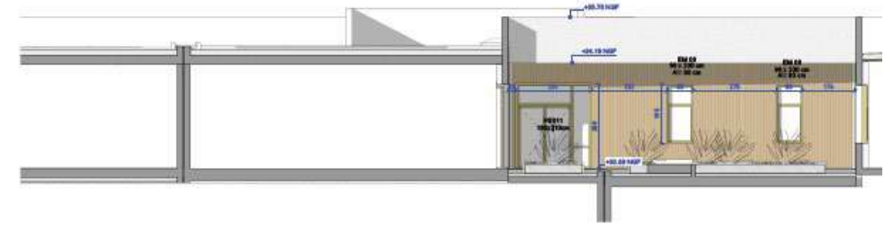
Façade Patio Nord _ APD Ech : 1 : 100
