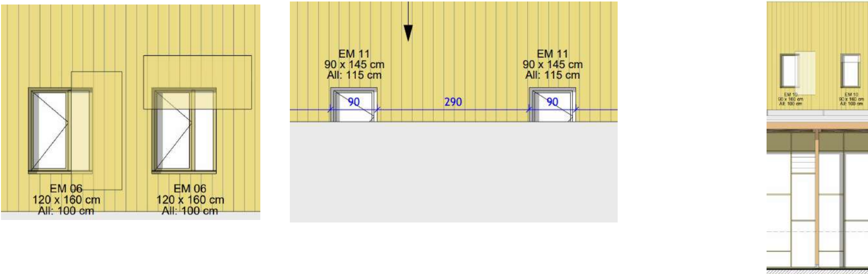
FACADE OUEST et EST BSO
