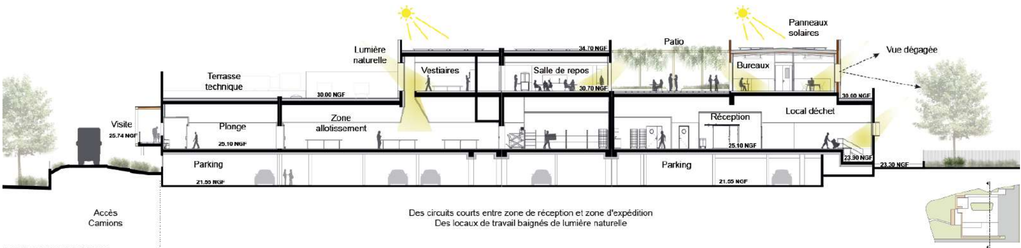
COUPE EST / OUEST Ergonomie de la BLTP
