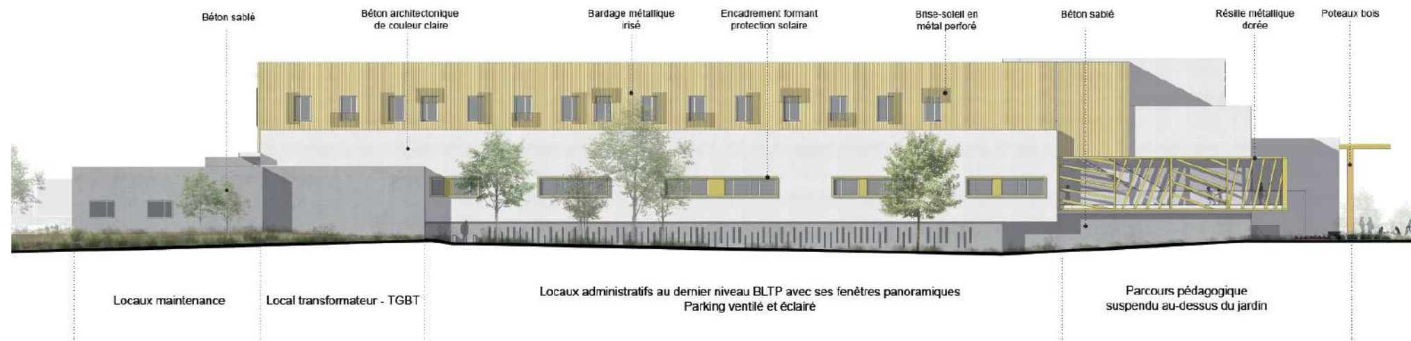
Façade Ouest
