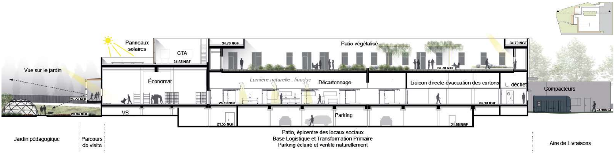
COUPE SUD / NORD Un patio à l'image d'une «place de village»
