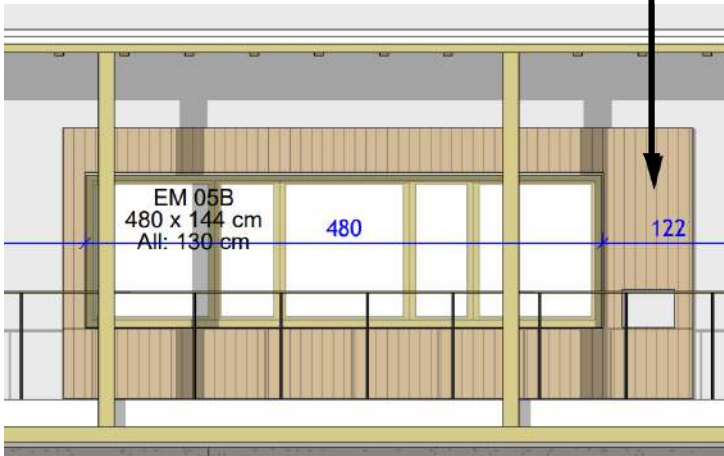
FACADE EST
