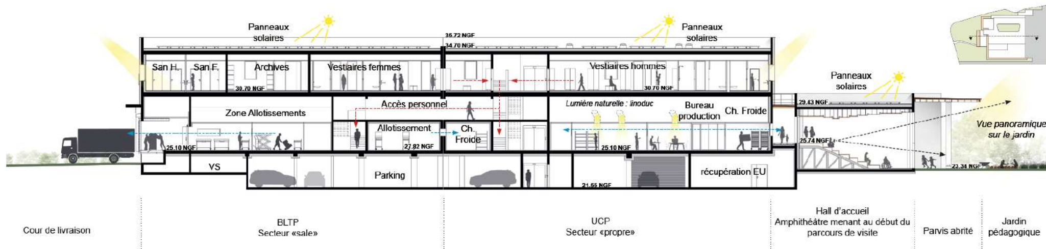
COUPE NORD / SUD Amphithéâtre : un lien entre la Terre et l'Assiette
