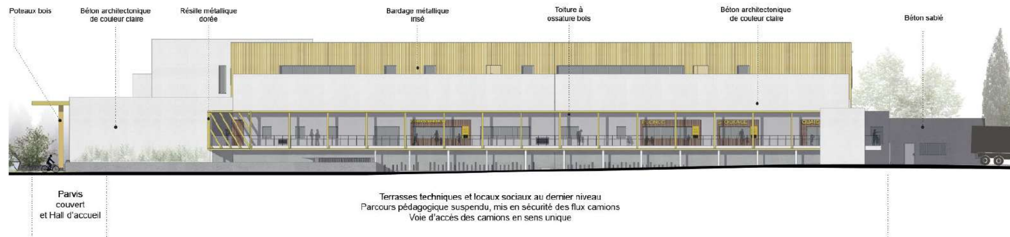
Façade Est
