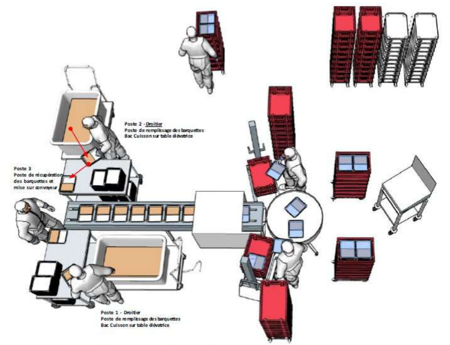
Conditionnement Barquettes avec deux Droitier au service
