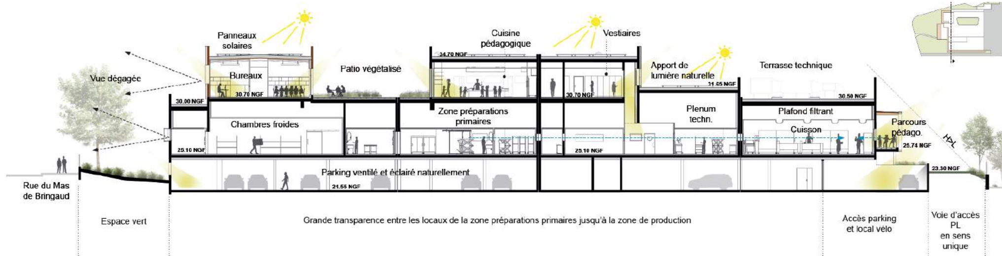
COUPE OUEST / EST Transparence du Process - Patio central
