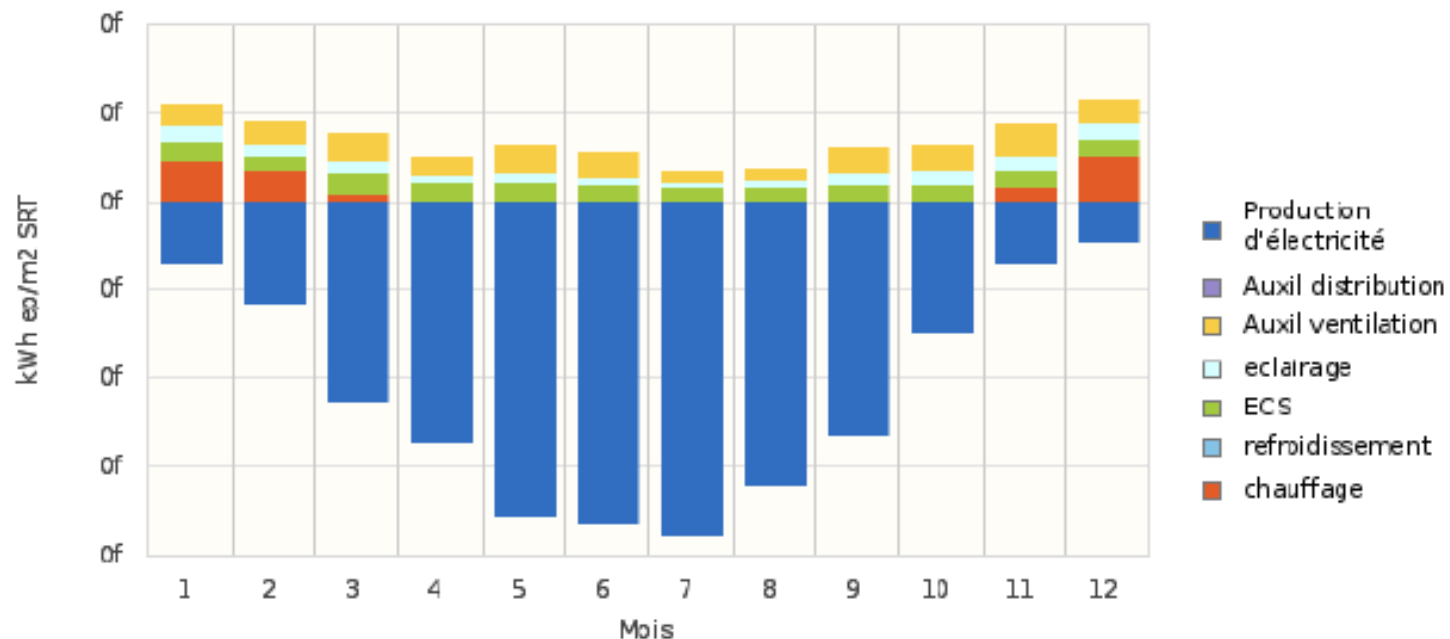
Consommation et production énergétique mensuelle en kWh ep /m 2
