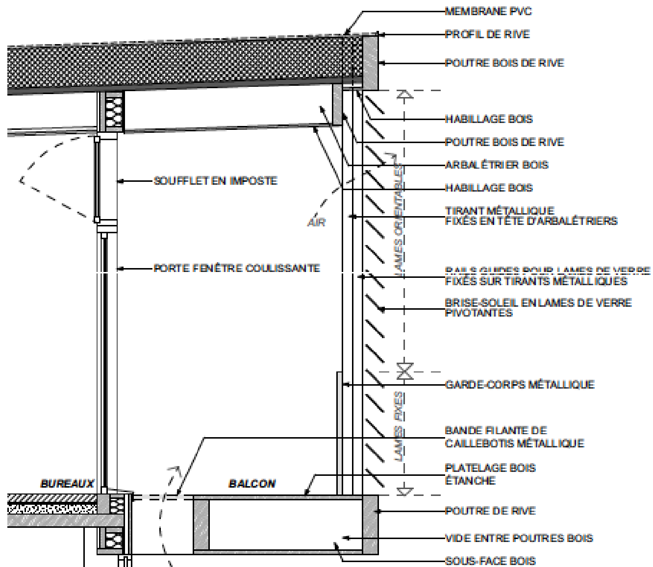
DÉTAIL 01 - BALCON
