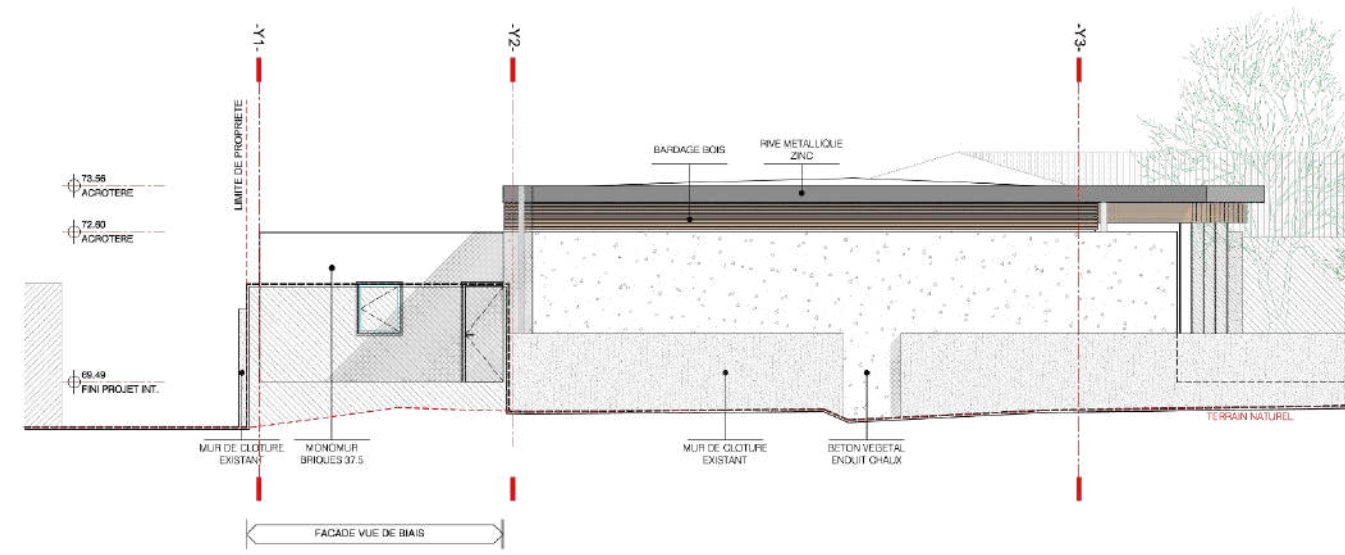
ELEVATION SUD
