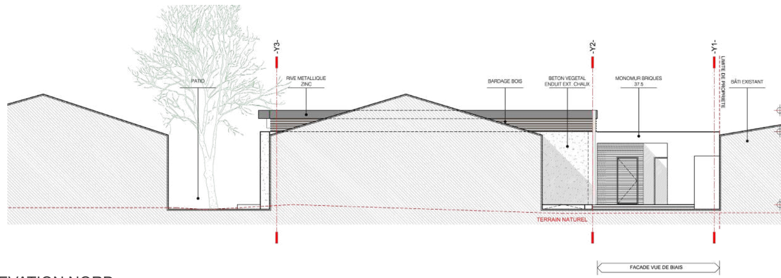
ELEVATION NORD
