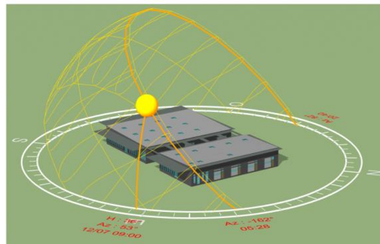
Position solaire et ombre sur la façade nord-ouest le 12/07 à 09h solaire
