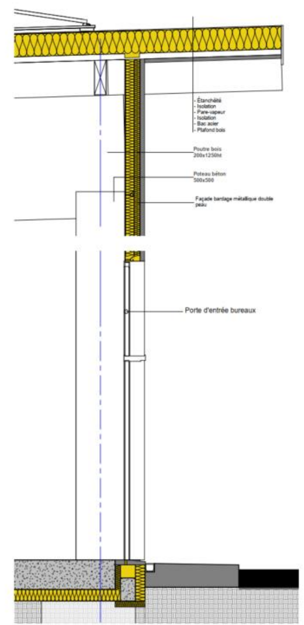
4 Coupe Façade - Portes bureaux 1 : 25
