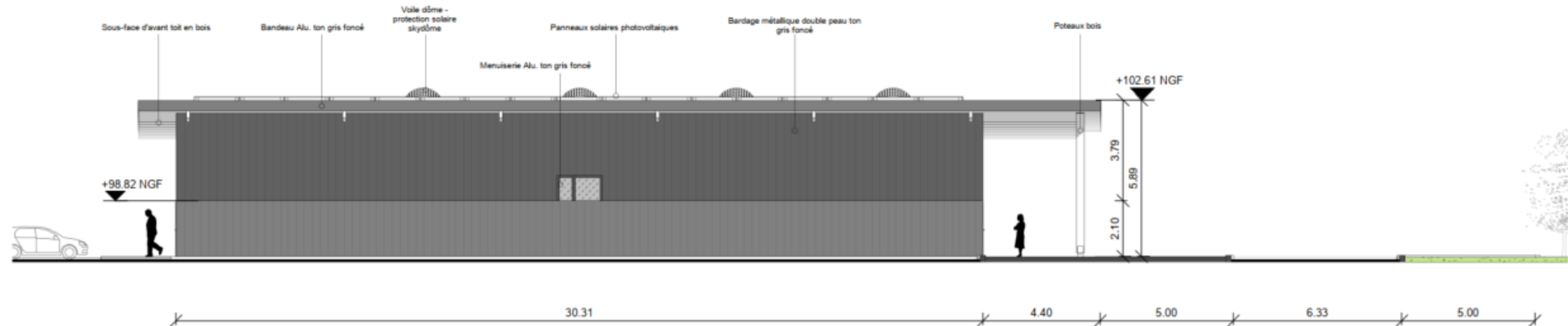
1 Elévation Sud 1 : 150
