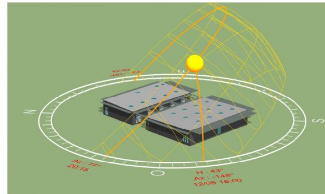
Position solaire et ombre sur la façade nord-ouest le 12/05 à 16h solaire
