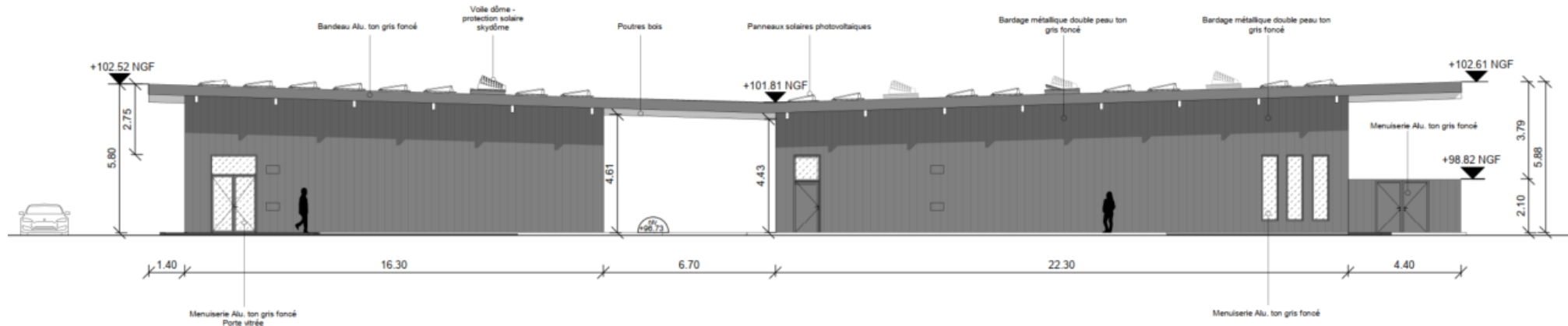
2 Elévation Ouest 1 : 150
