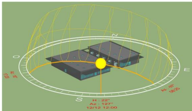
Position solaire et ombre sur la façade sud-est le 12/12 à 12h solaire
