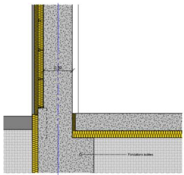
2 Coupe Façade - Poteaux - Rue intérieur / Salle de vente 1 : 25
