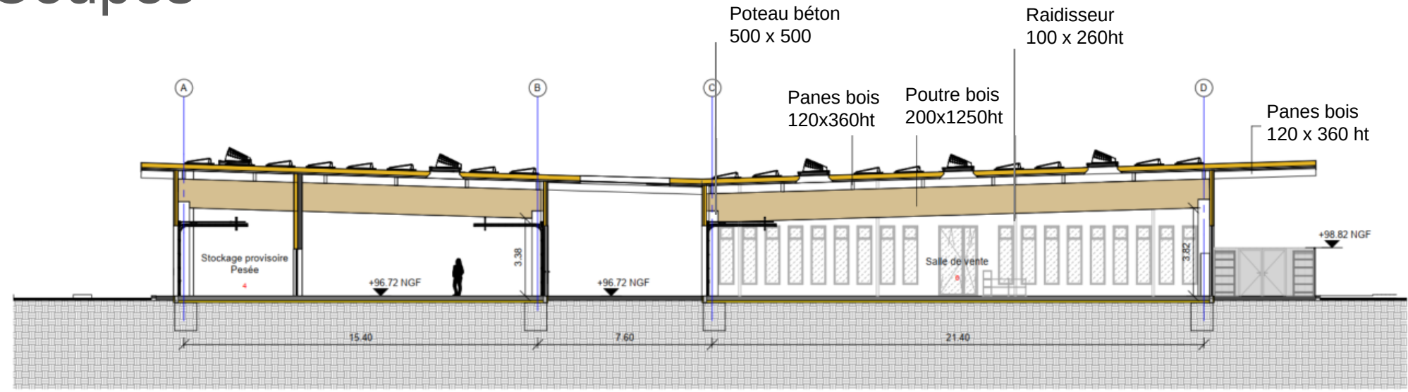
1 Coupe longitudinale 1 : 150
