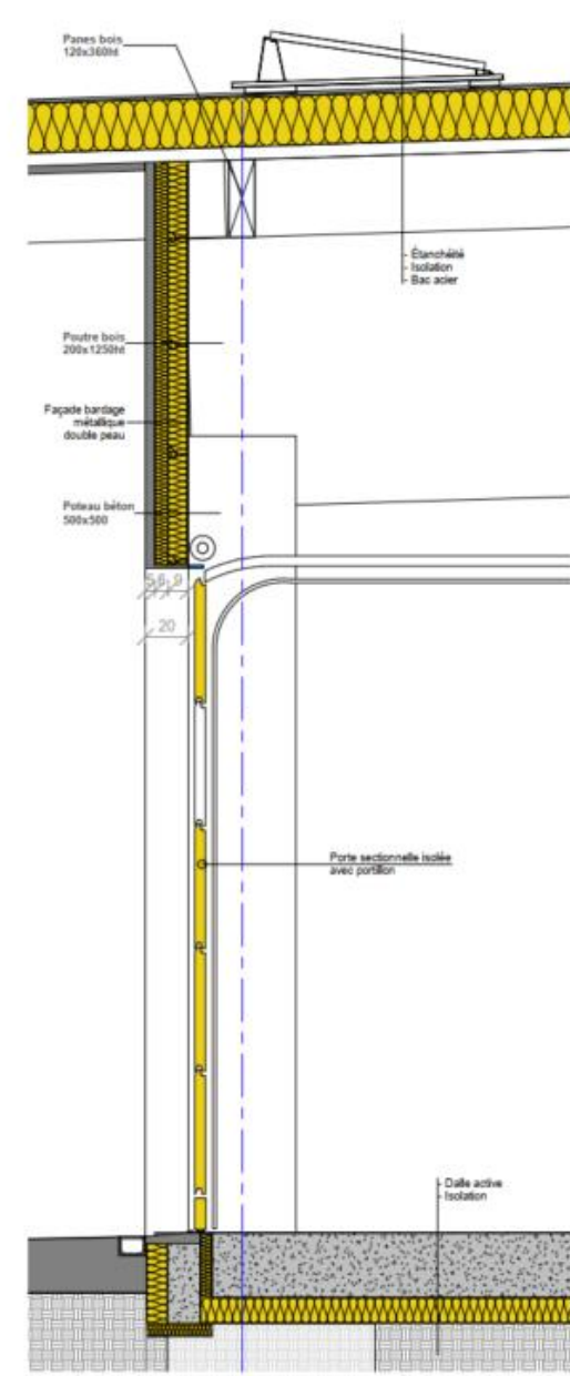
3 Coupe Porte Sectionnelle Ateliers - Rue intérieur 1 : 25
