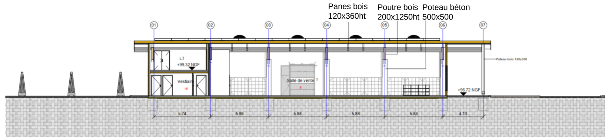
2 Coupe transversale 1 : 150
