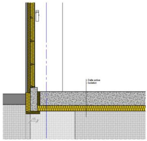
1 Coupe Façade - Rue intérieur / Salle de vente 1 : 25
